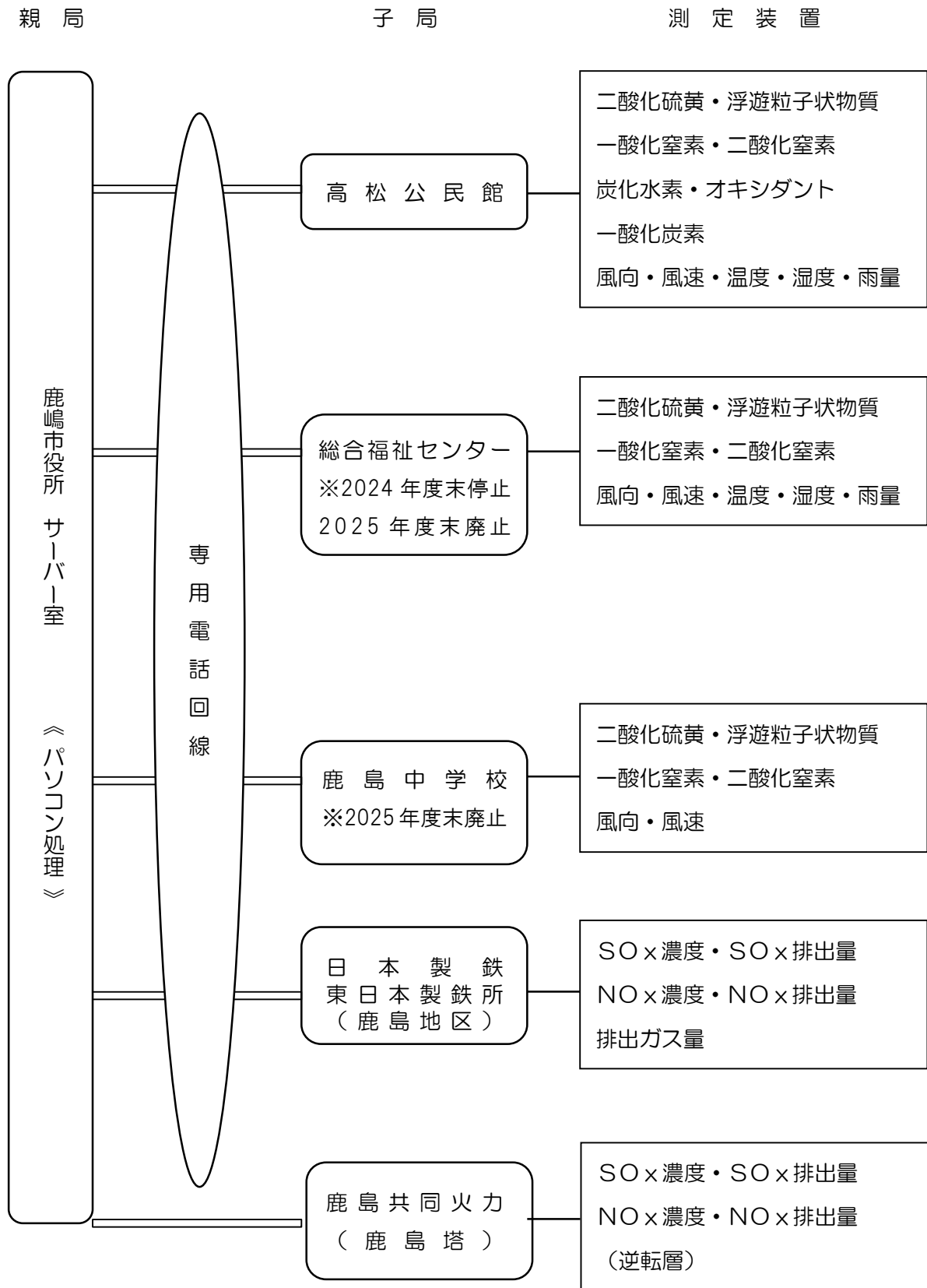
図1-1-2 大気汚染常時監視テレメータシステム 構成・測定項目
