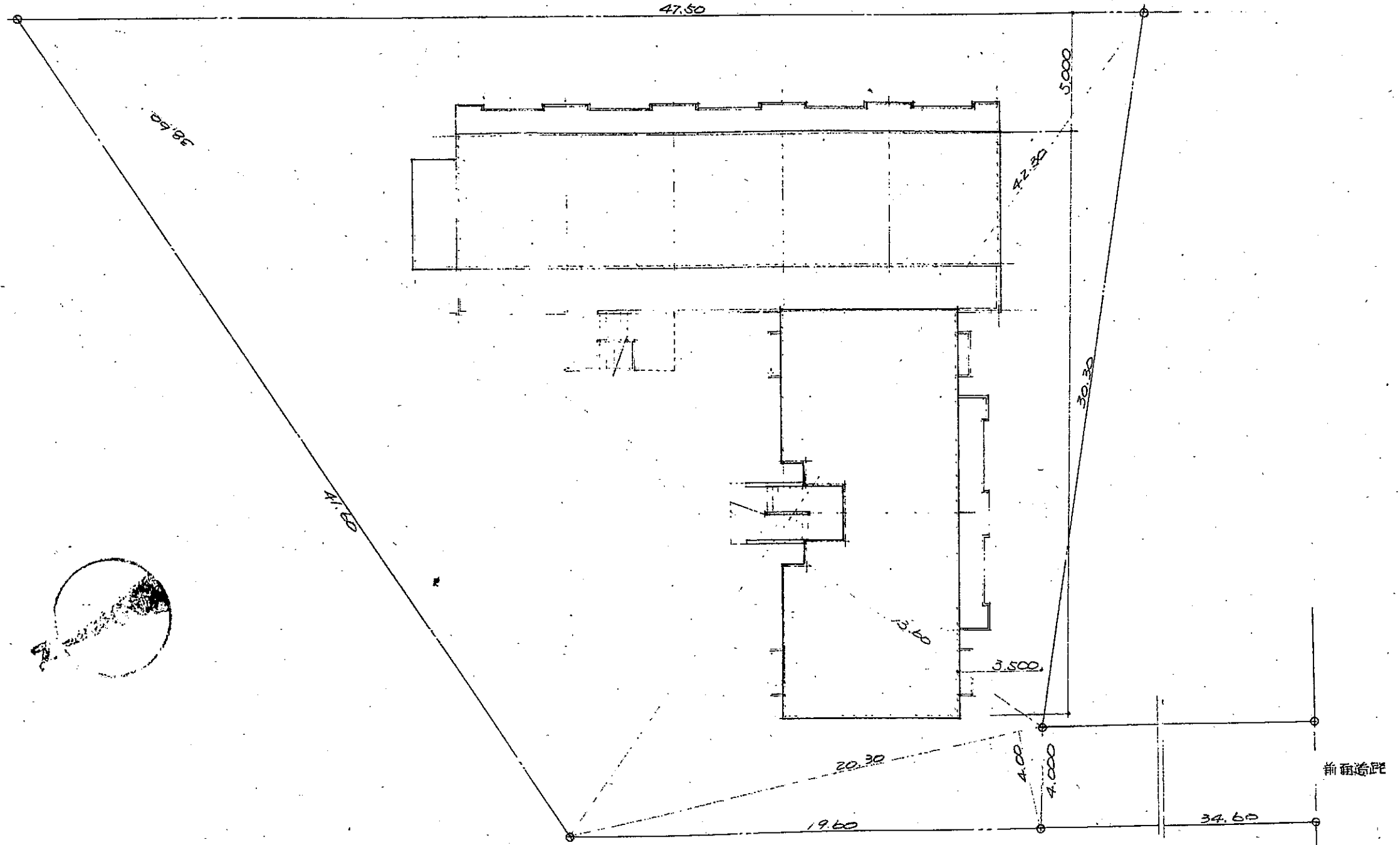
配置图 1:200
